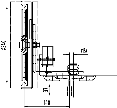
对称装配
