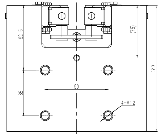
视图 A
