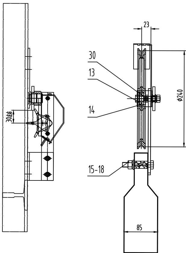
OX300 (240-135/220-27) 涨紧装置 (本件可左右对称使用)
