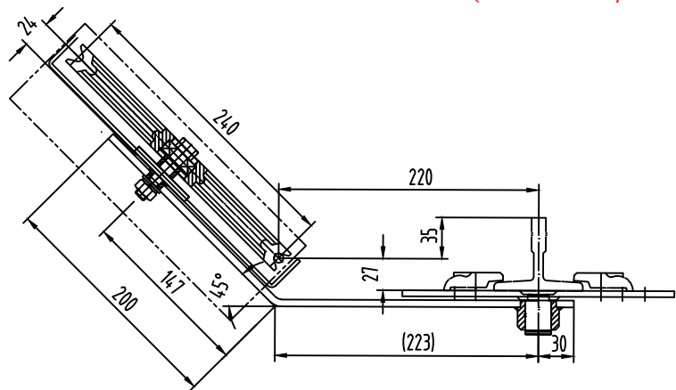
OX300 (240-135/220-27) 涨紧装置 (本件可左右对称使用)
