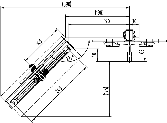
一次性用图(左右对称装配各一)
