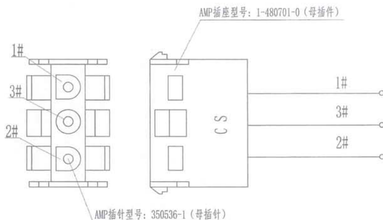
接插件接头热缩管示意图
