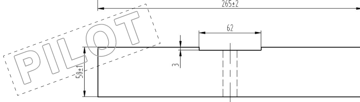
配重块图纸（铸铁）附图
