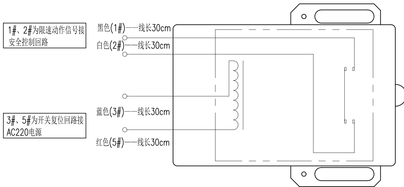
线号示意 (接插件时)
