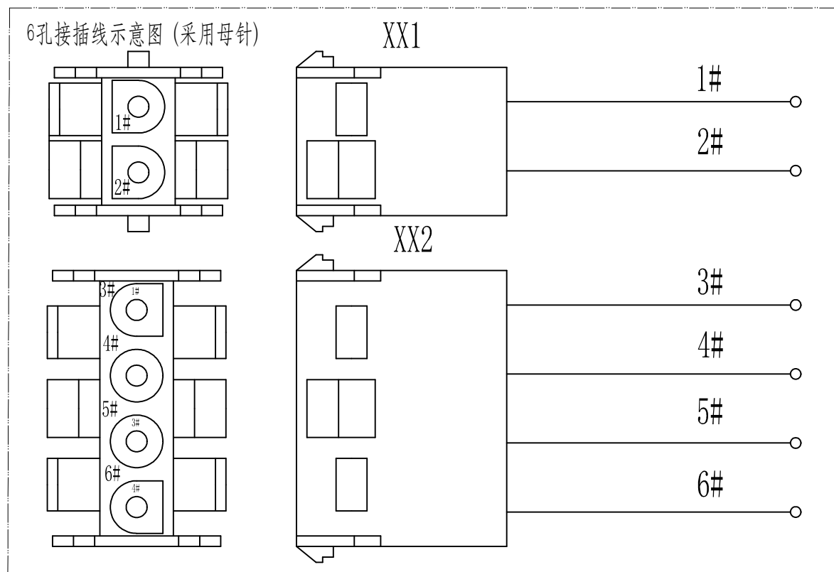
线号示意 (接插件时)
