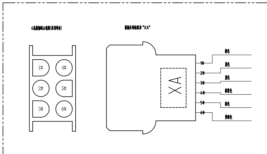
线号示意 (接插线时)
