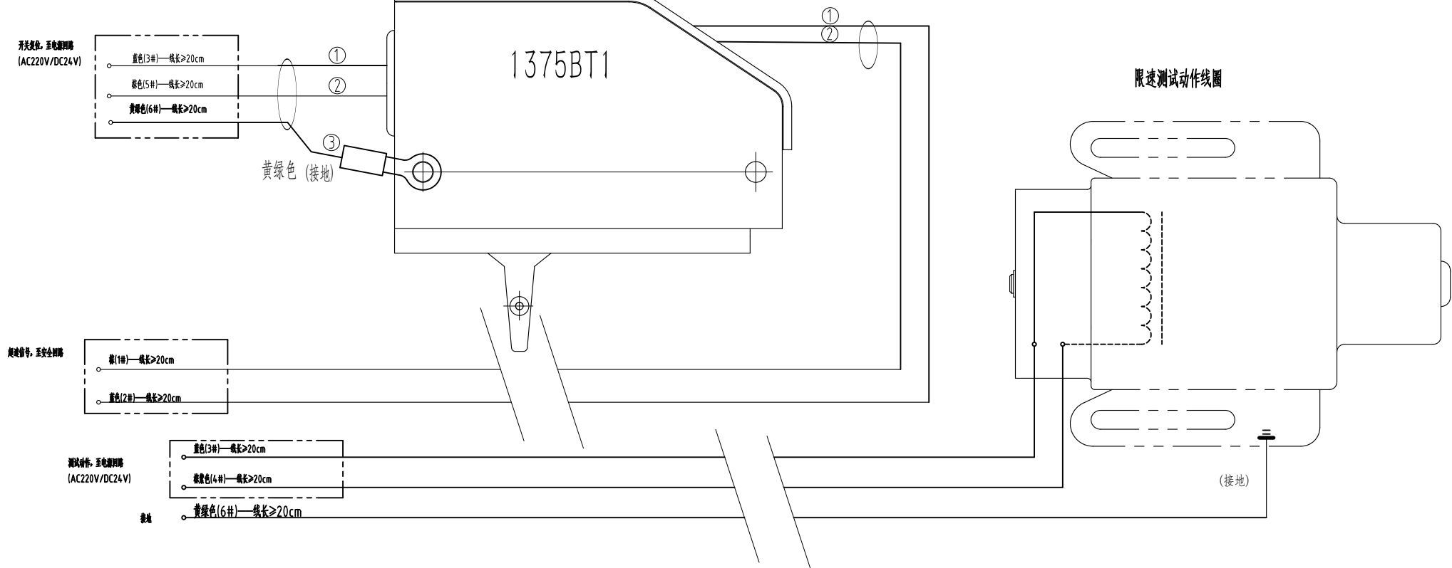
线号示意 (接插线时)
