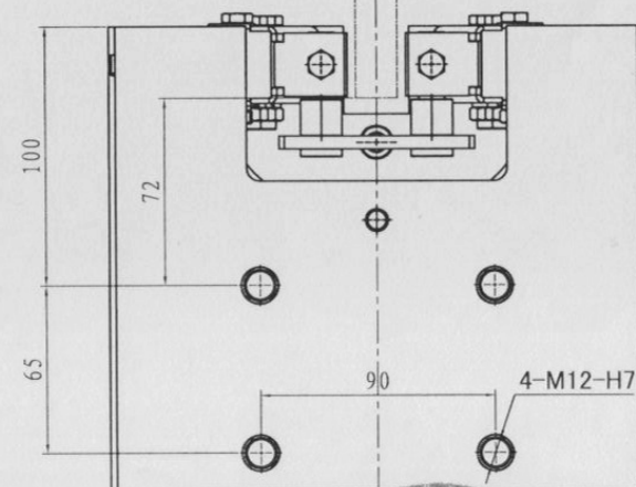
视图 A
