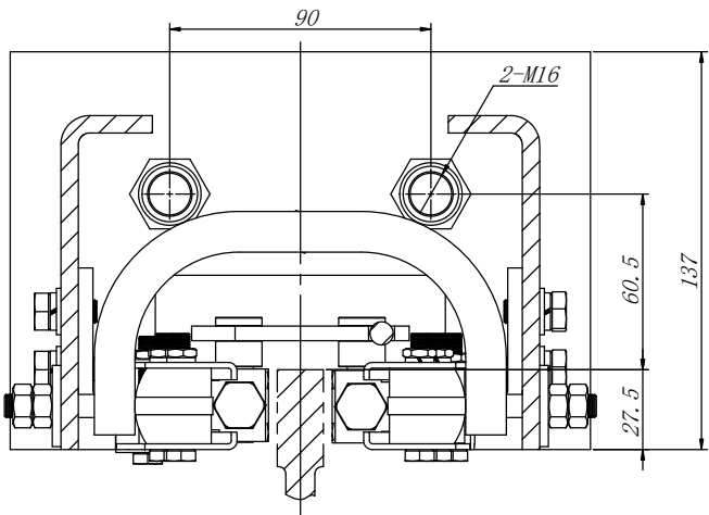
剖面 A-A
