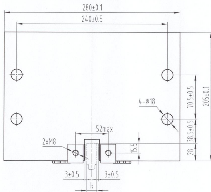
(安全钳安装面)
