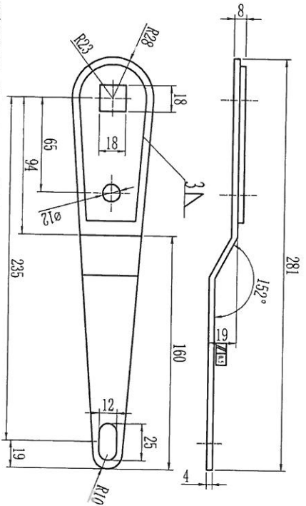
摇臂提拉组件 2件 MSA3H519001 (特检自制)
